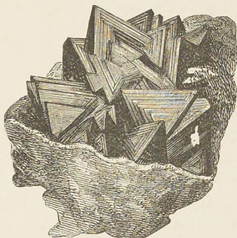
BLENDE.
